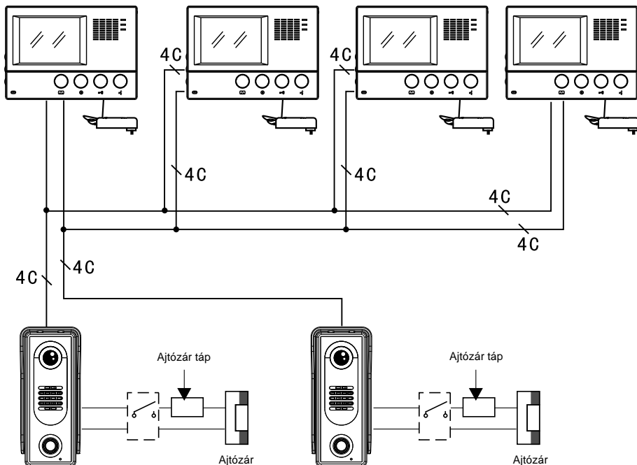
1-es kültéri kaputelefon
